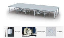
气浮台板 Air Flotation Table
